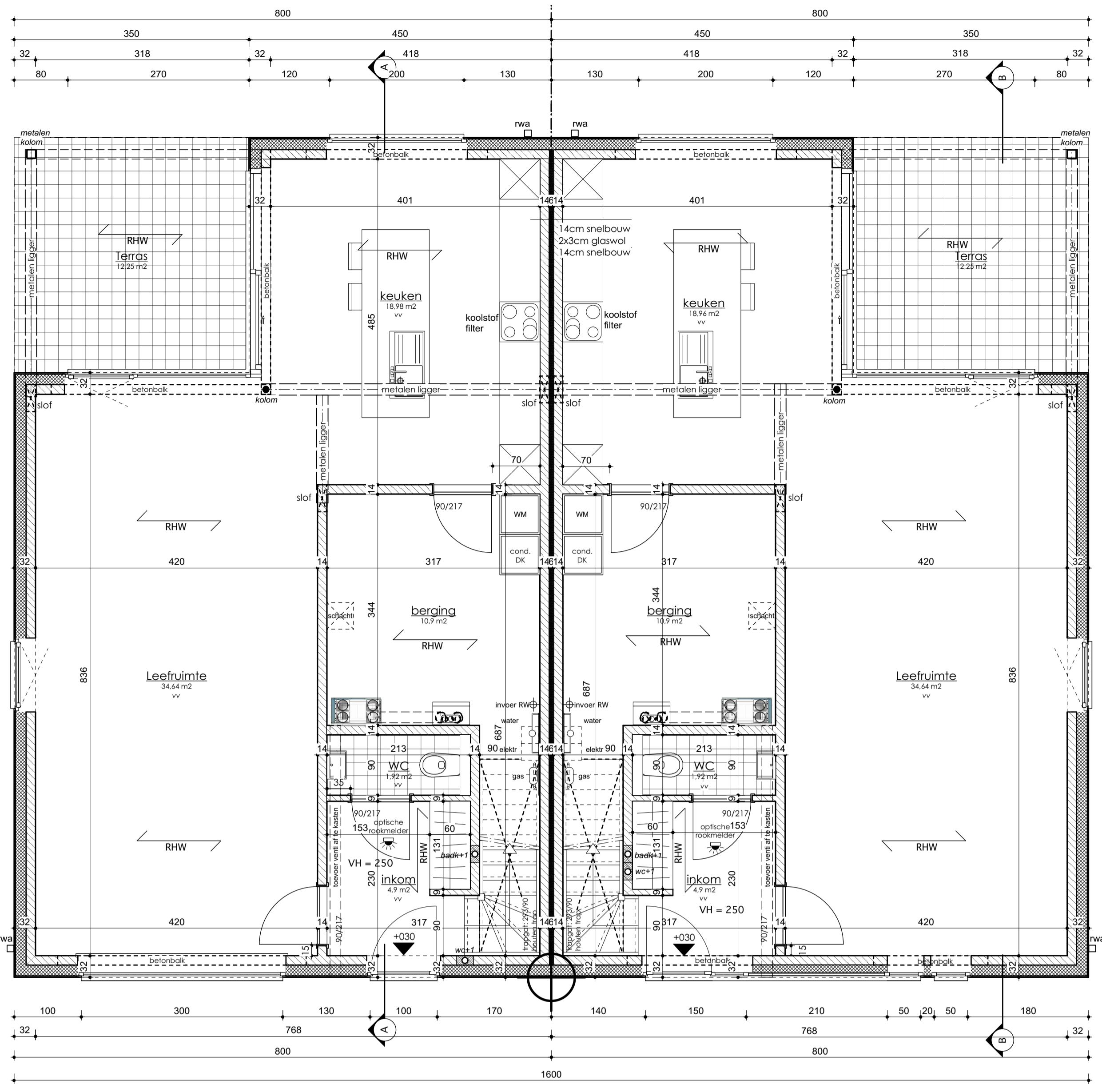
Gelijvloers Schaal: 1:50
