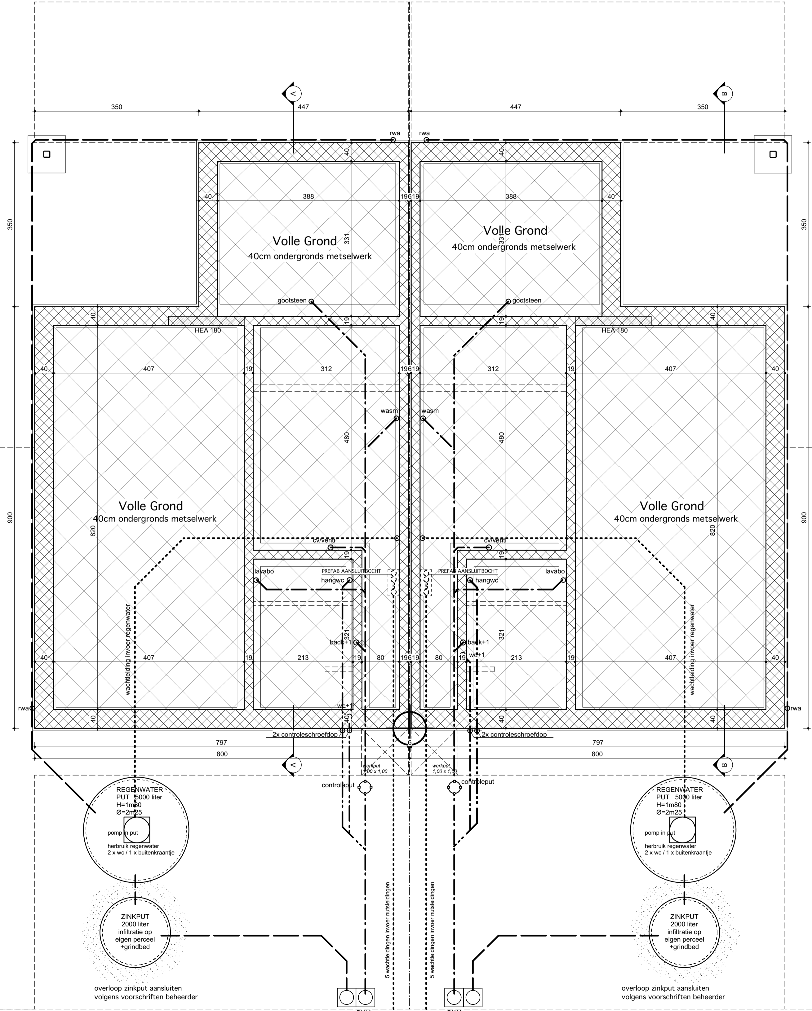
Schaal: 1:50 Funderings- en Rioleringsplan
